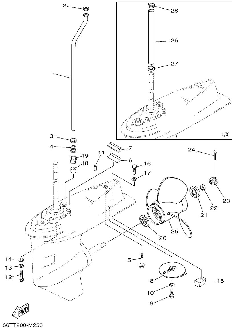
66TT200-M250
